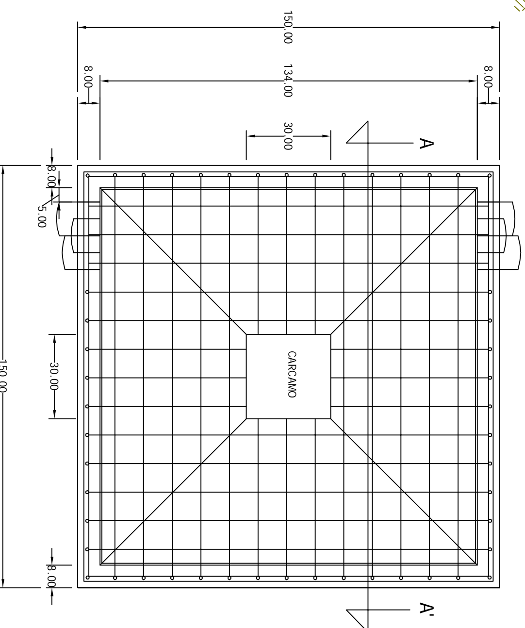
PLANTA PISO
