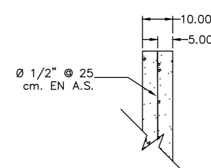
DETALLE 1
