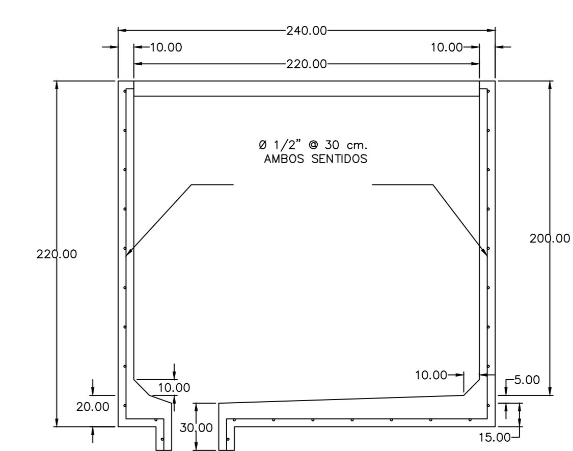
PARA NIVEL FREÁTICO BAJO SECCIÓN CORTE A-A'
