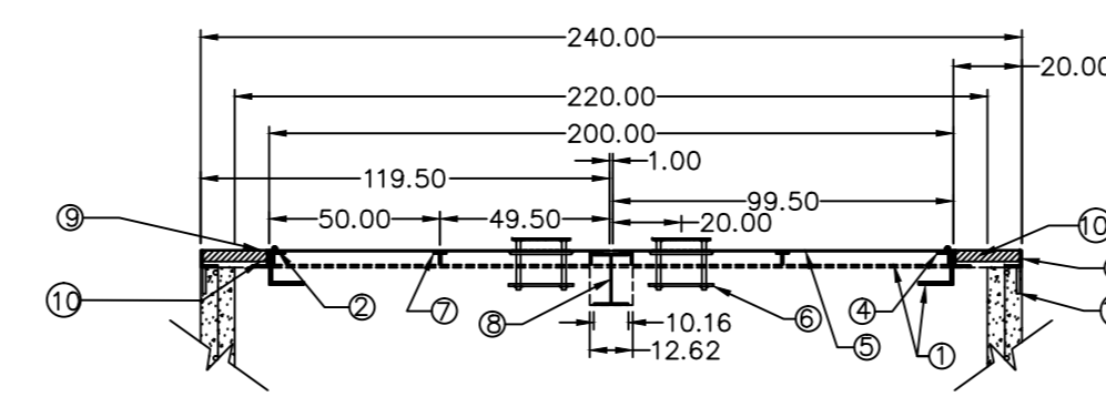
PLANTA SECCIÓN CORTE C-C'
