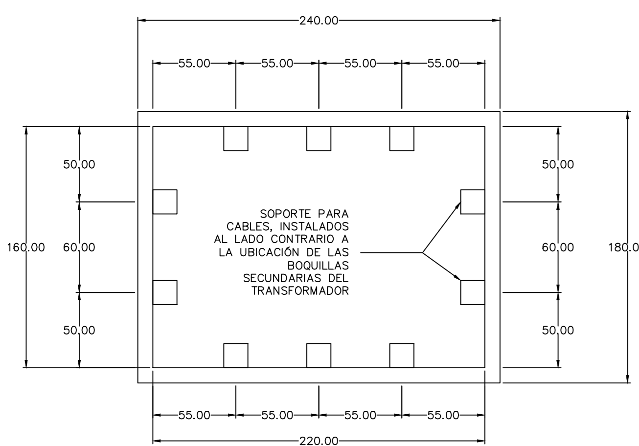
CORREDERAS PARA SOPORTE DE CABLES
