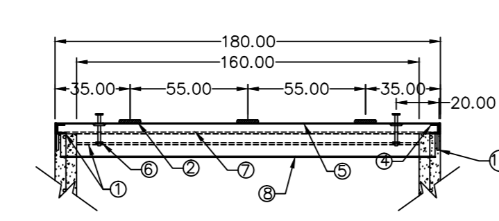
PLANTA SECCIÓN CORTE D-D'
