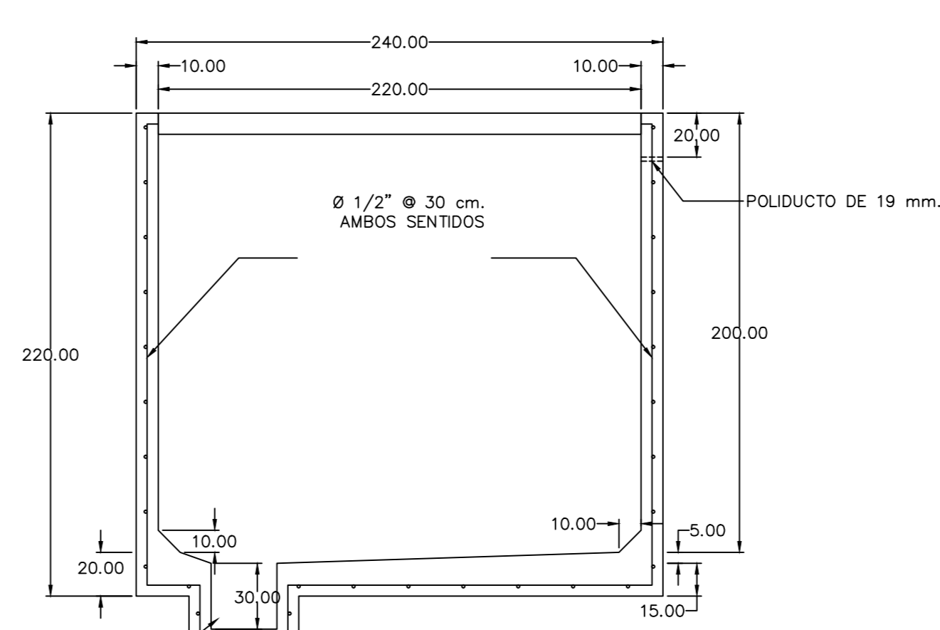
PARA NIVEL FREÁTICO ALTO SECCIÓN CORTE A-A'
