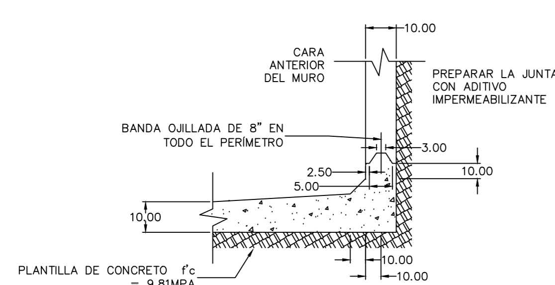
DETALLE 2
