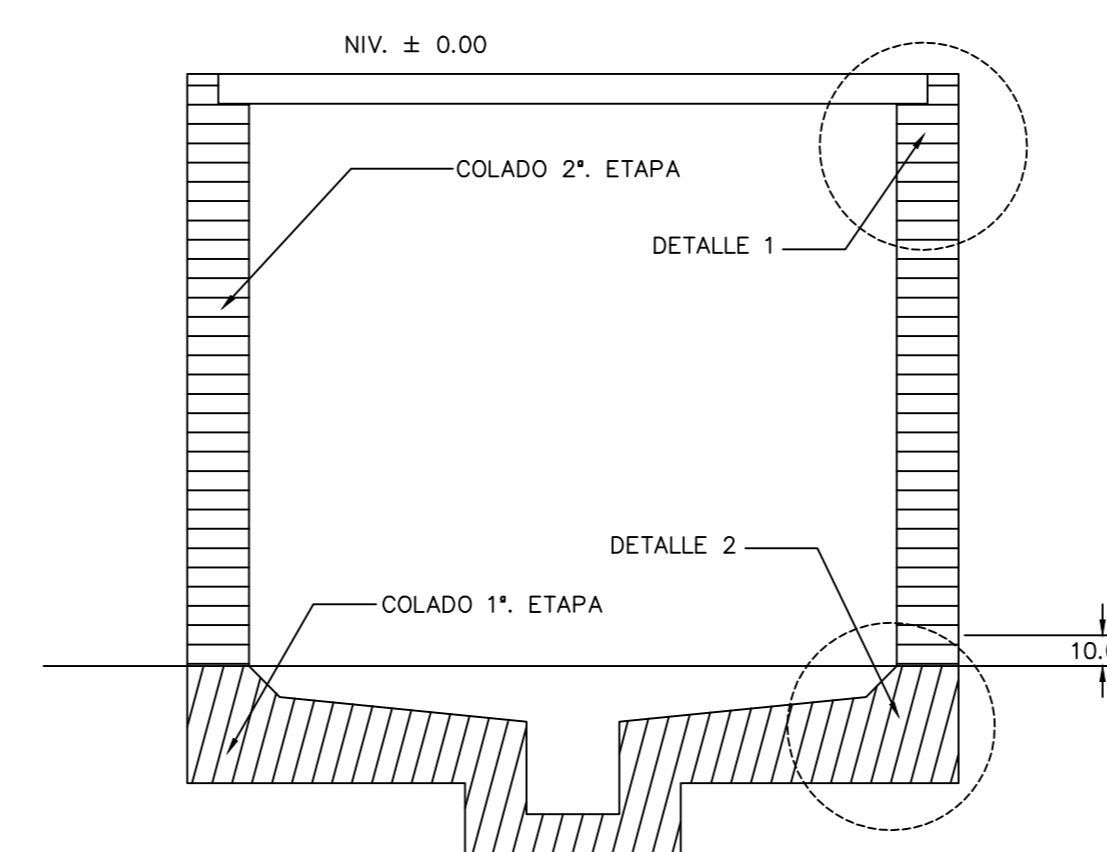
ETAPAS DE COLADO
