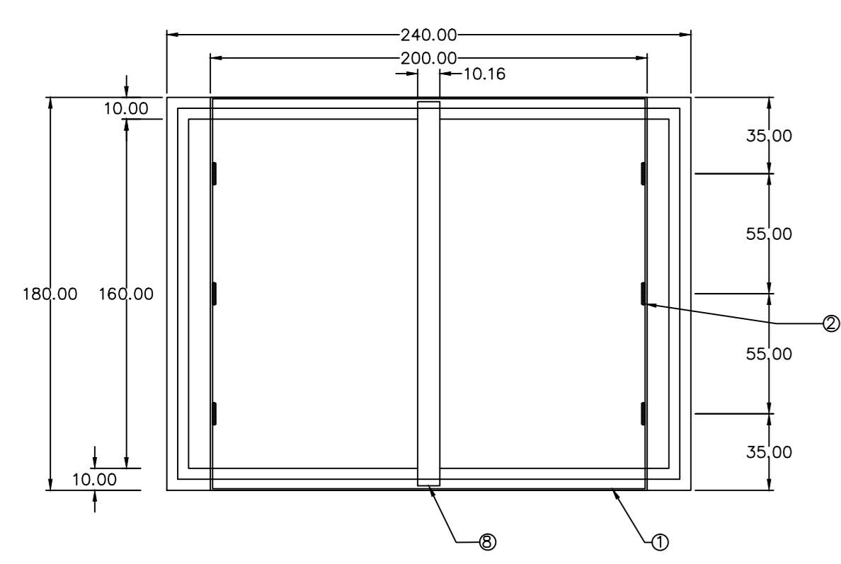
PLANTA MARCO Y BÓVEDA
