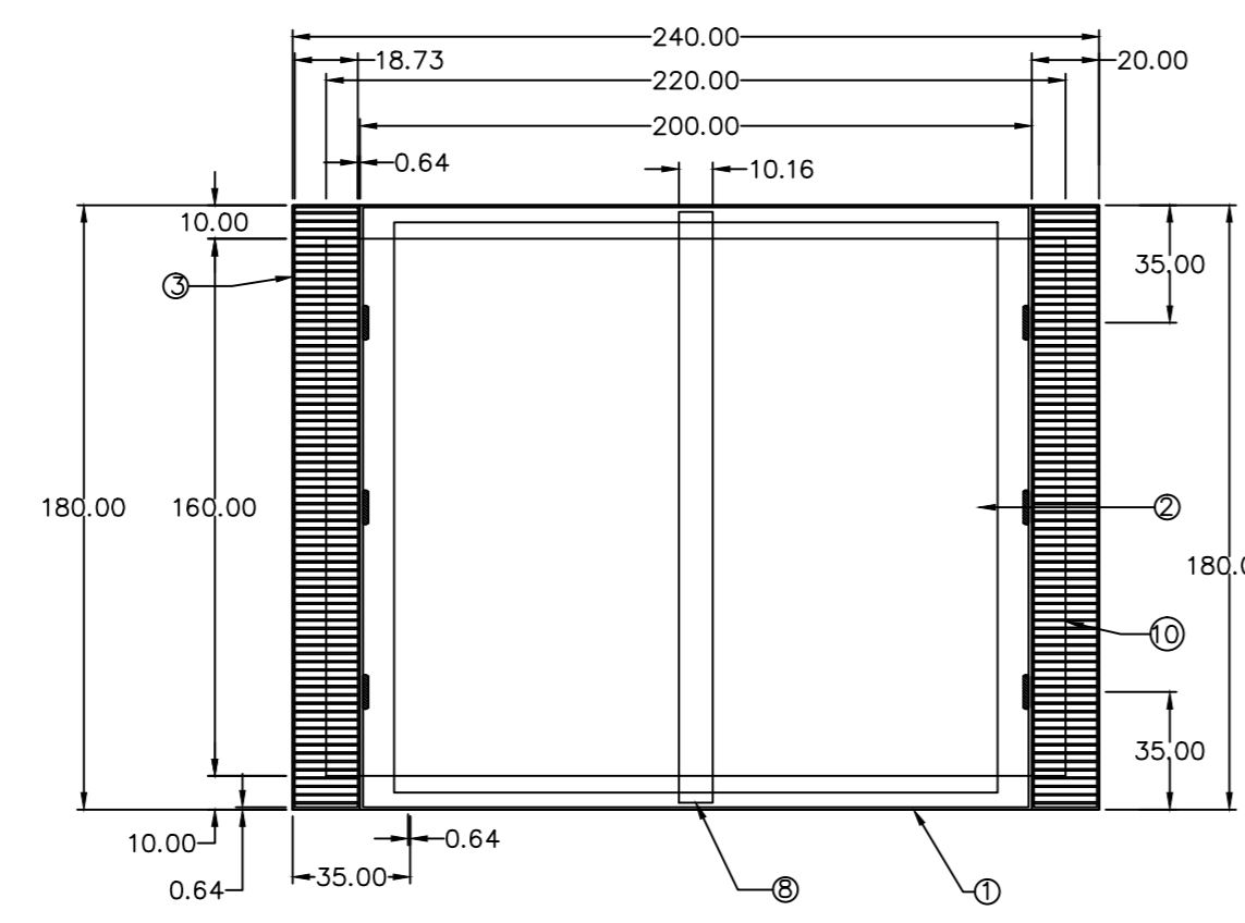
PLANTA MARCO, REFUERZOS Y REJILLA
