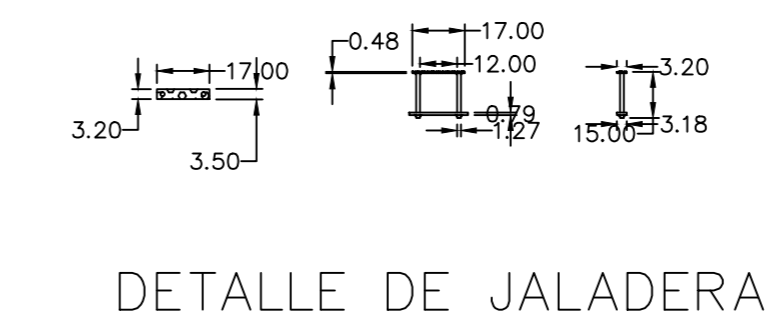
DETALLE DE JALADERA
