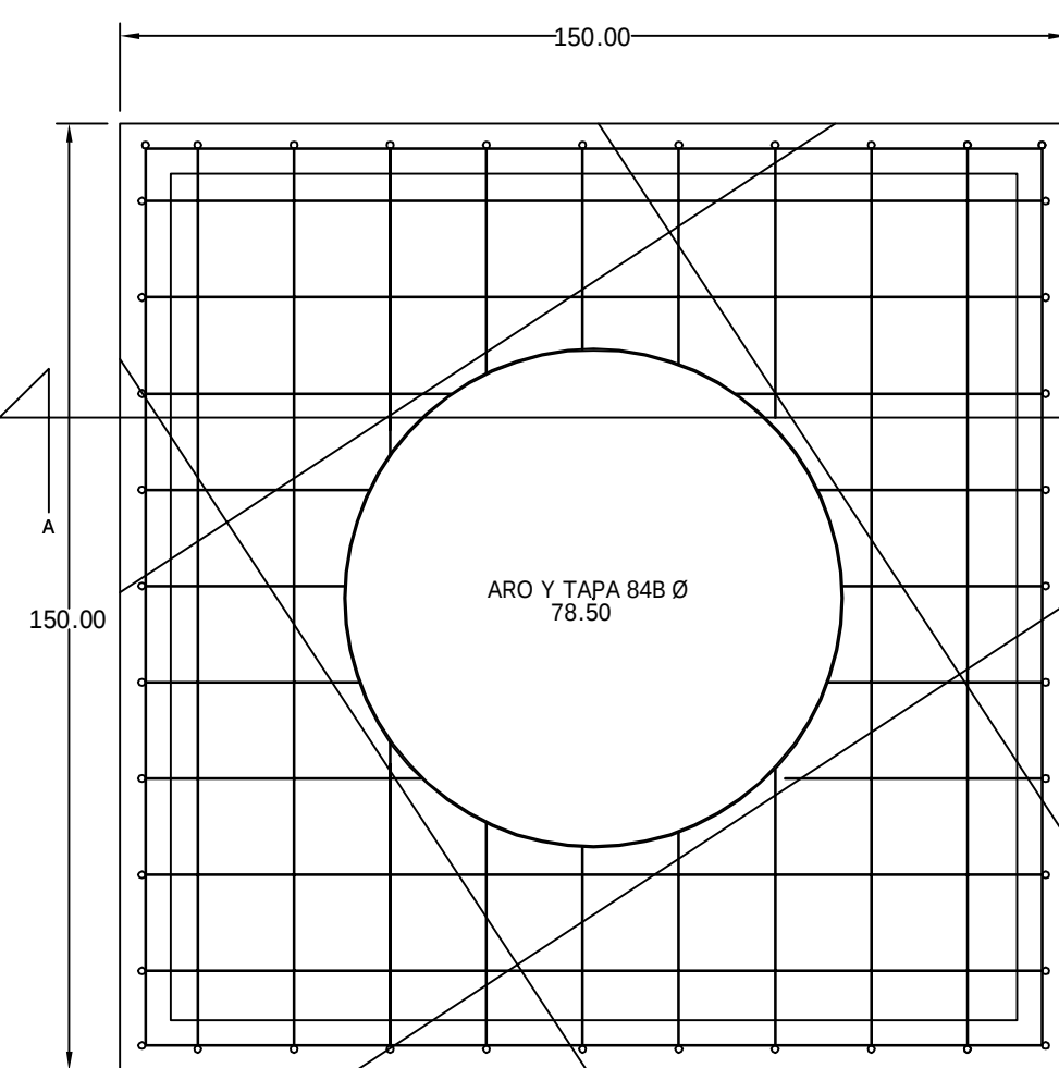
PLANTA PISO
