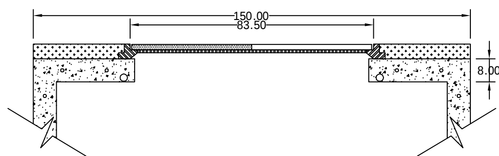
DETALLE COLOCACION ARO Y TAPA
