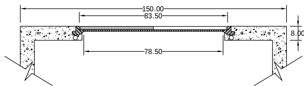
DETALLE COLOCACION ARO Y TAPA
