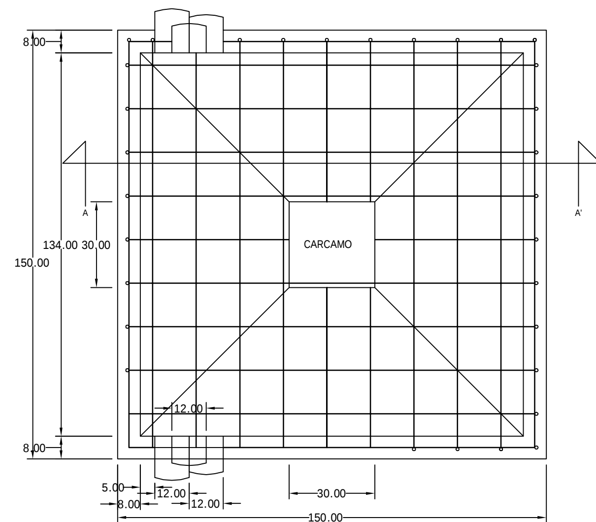
PLANTA PISO
