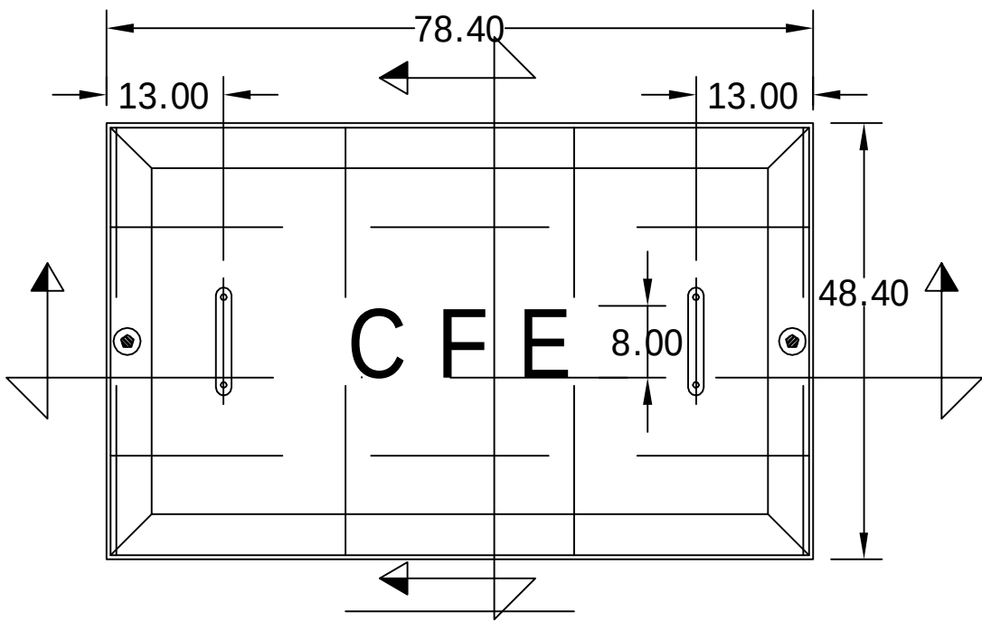
PLANTA TAPA
