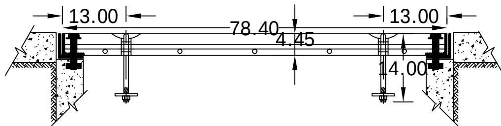
DETALLE TAPA: CORTE C-C'
