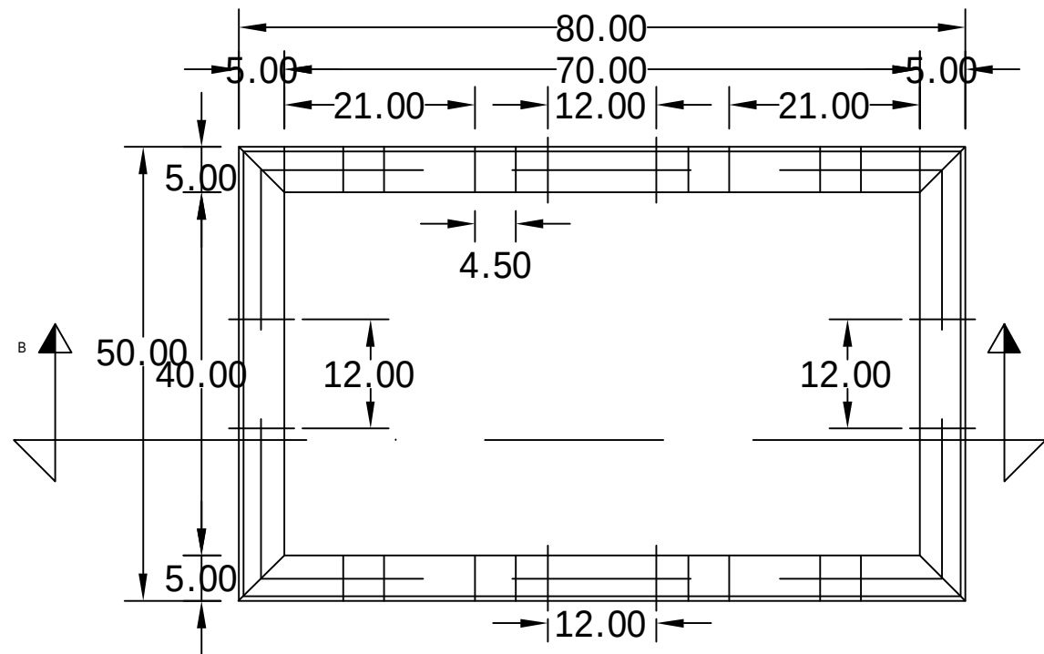
PLANTA REGISTRO SIN FONDO
