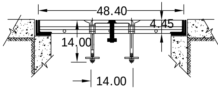
DETALLE TAPA: CORTE D-D'
