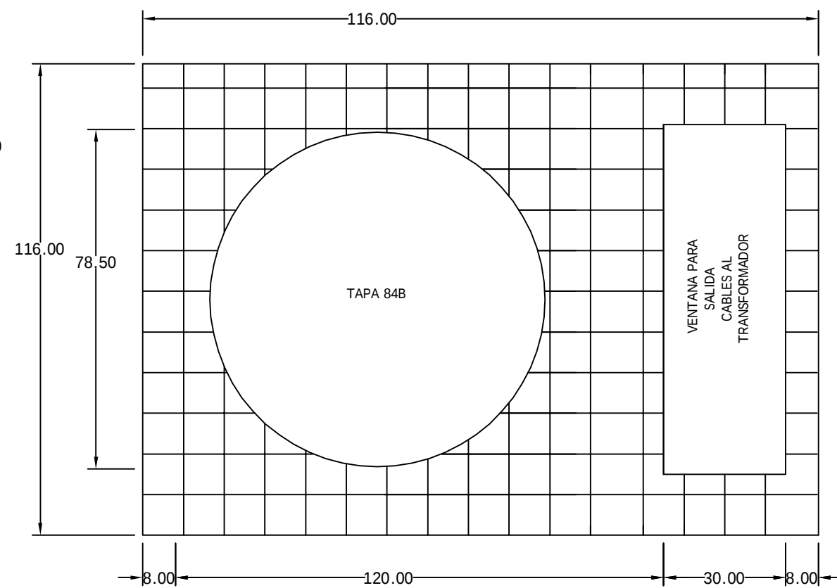
PLANTA BASE PARA TRANSFORMADOR Y REGISTRO TIPO 3 EN BANQUETA
