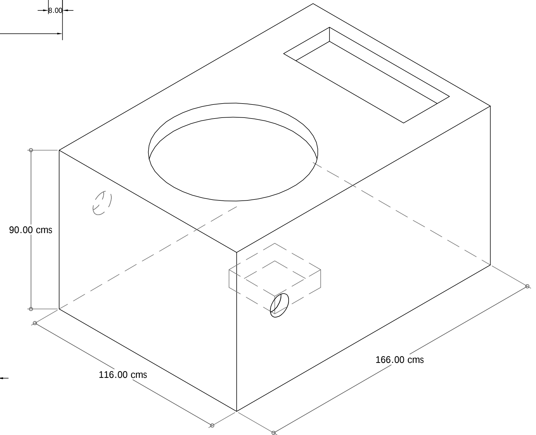
PLANTA BASE PARA TRANSFORMADOR Y REGISTRO TIPO 3 EN BANQUETA
