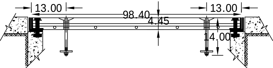
DETALLE TAPA: CORTE C-C'
