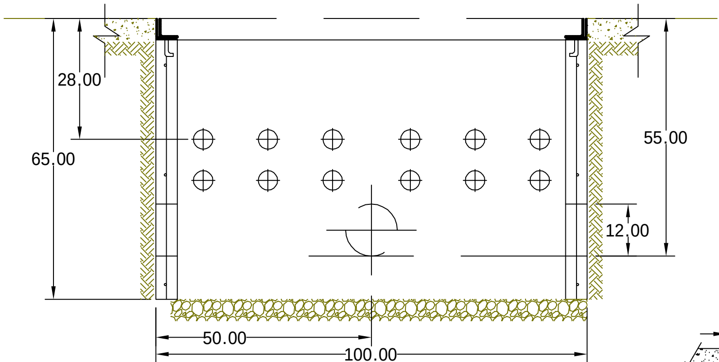
REGISTRO SIN FONDO PARA NIVEL FREATICO BAJO
