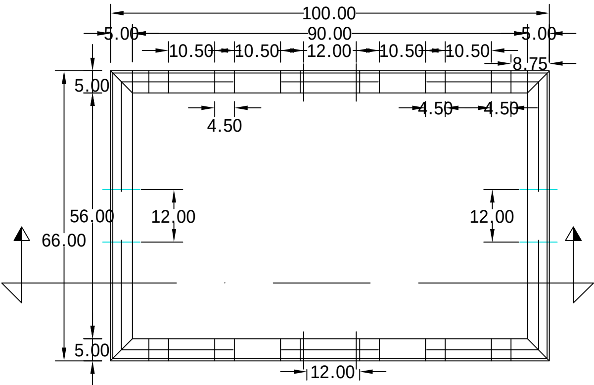
PLANTA REGISTRO SIN FONDO
