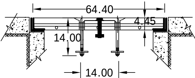
DETALLE TAPA: CORTE D-D'
