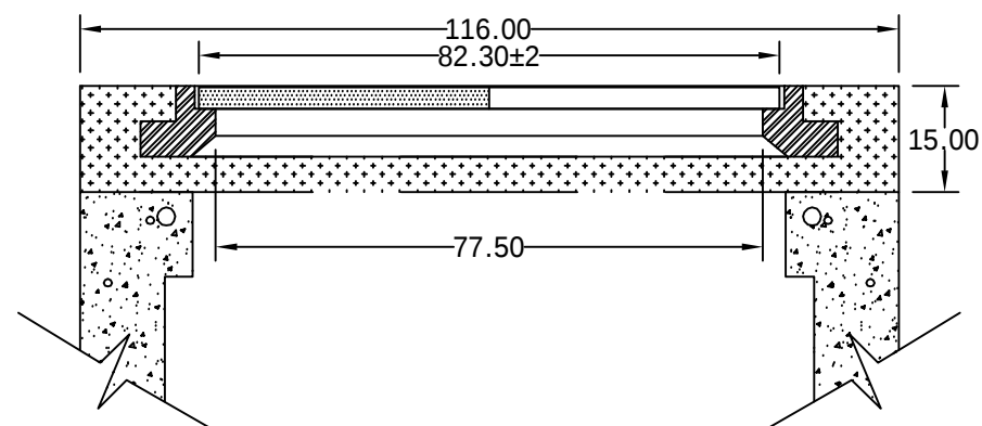
DETALLE COLOCACION MARCO Y TAPA
