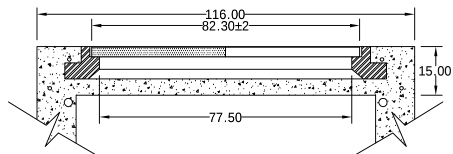
DETALLE COLOCACION MARCO Y TAPA
