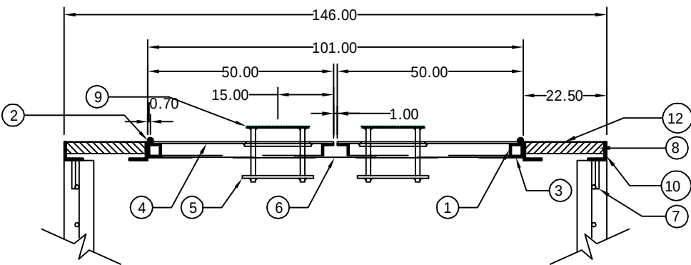
CORTE TAPA D-D'
