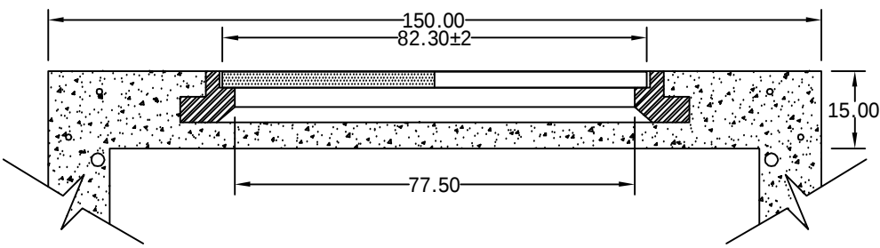
DETALLE COLOCACION MARCO Y TAPA
