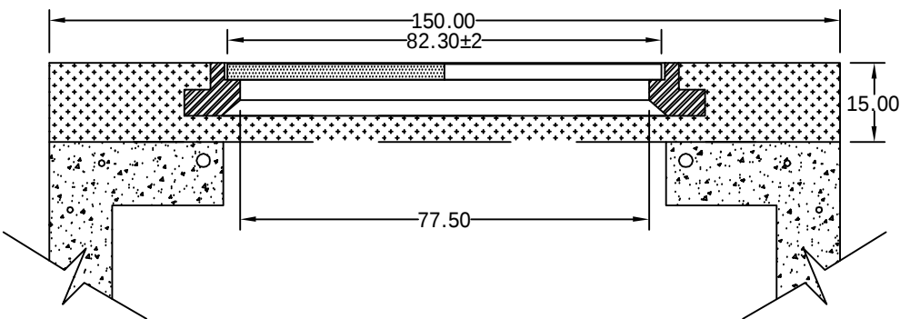
DETALLE COLOCACION MARCO Y TAPA
