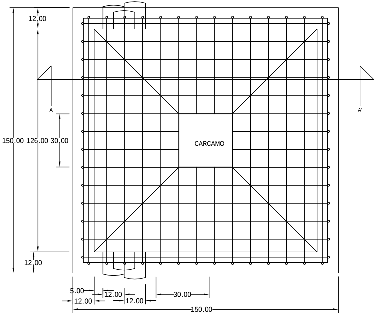
PLANTA PISO
