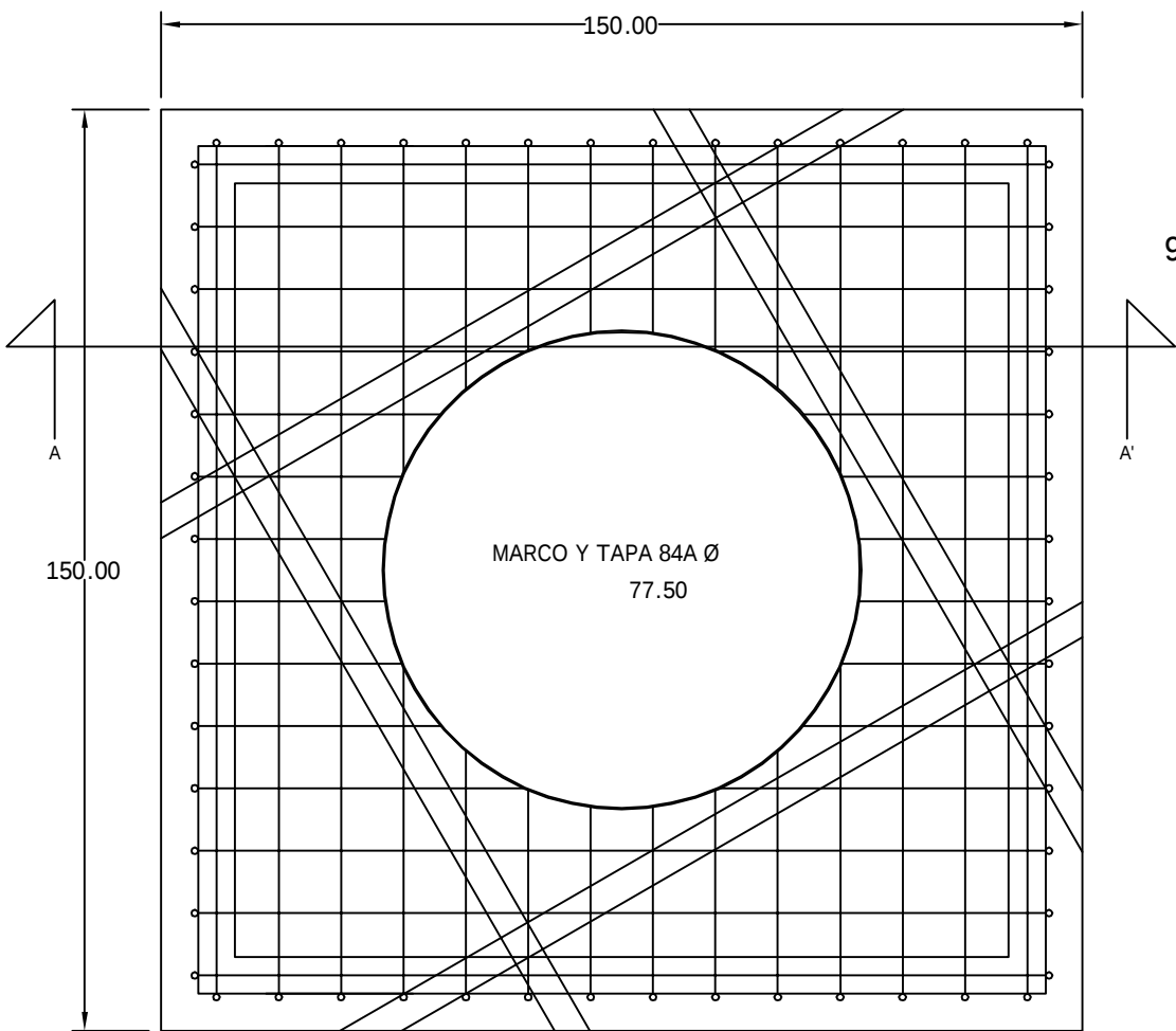
PLANTA PISO
